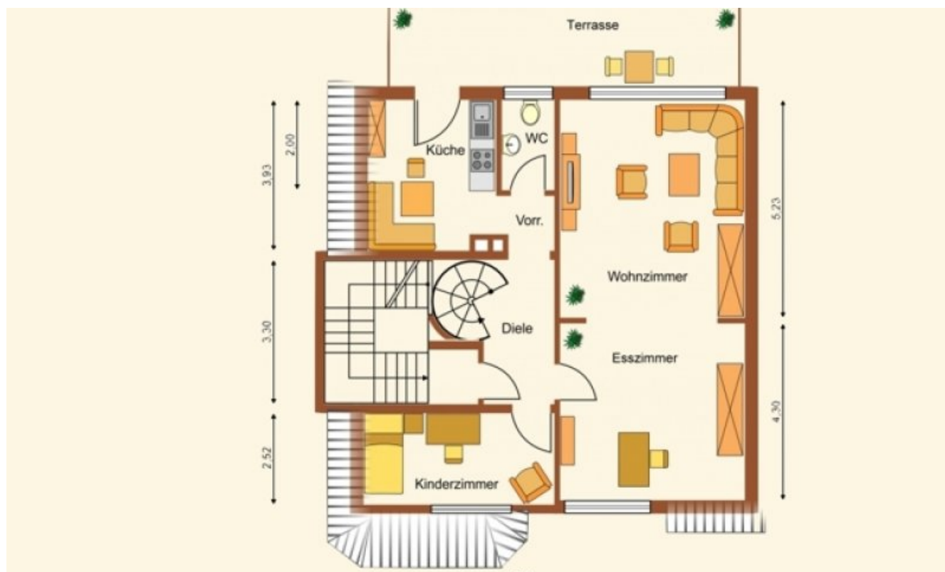
Obergeschoß (Grundriss)
